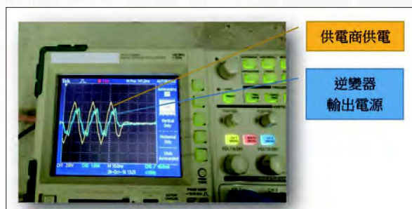
圖 3：以視波器測試及記錄逆變器的「防孤島」功能
