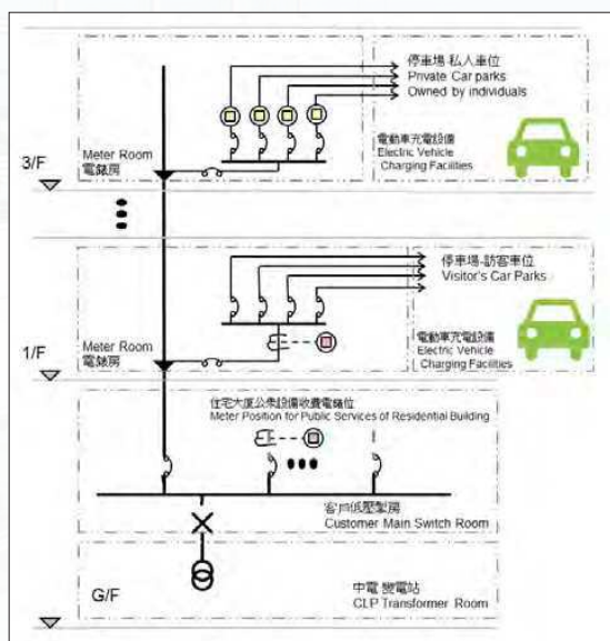
(圖一) 一般大廈安裝電動車供電設施
