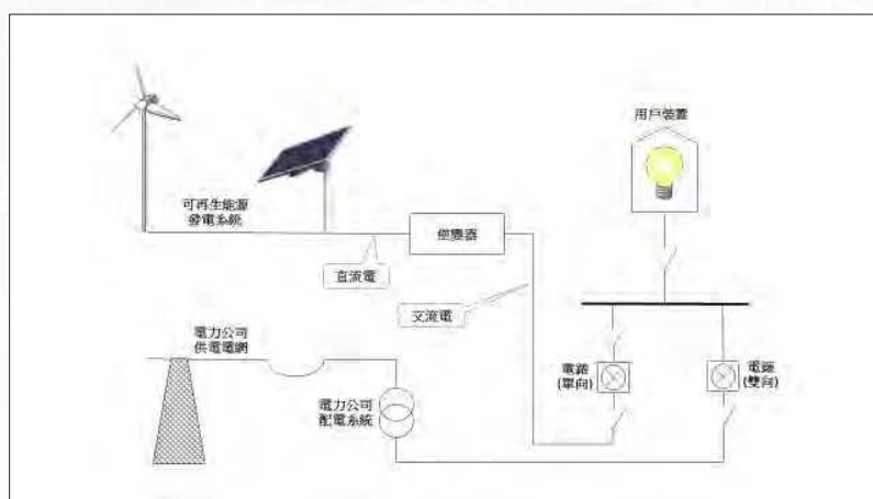
圖 1：可再生能源發電系統接駁至電網的一般示意圖
